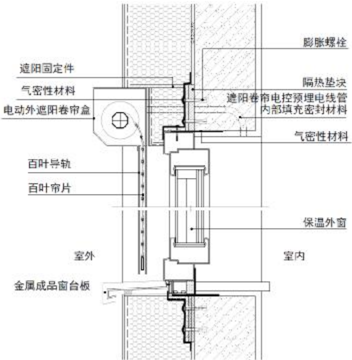
图 8 活动外遮阳示意图
