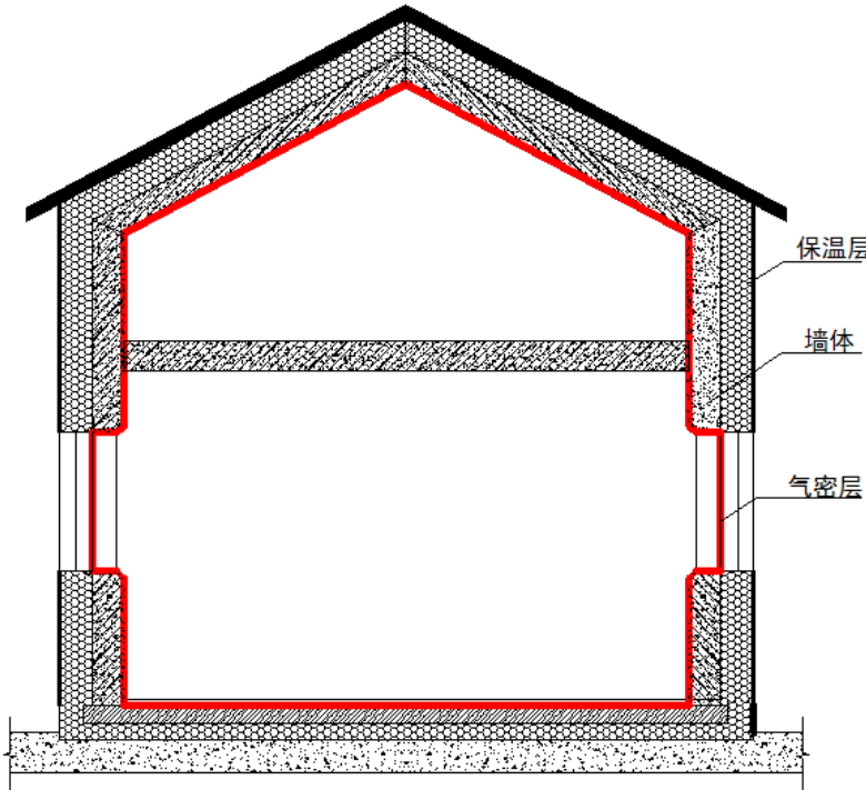
图 16 气密层标注示意图
