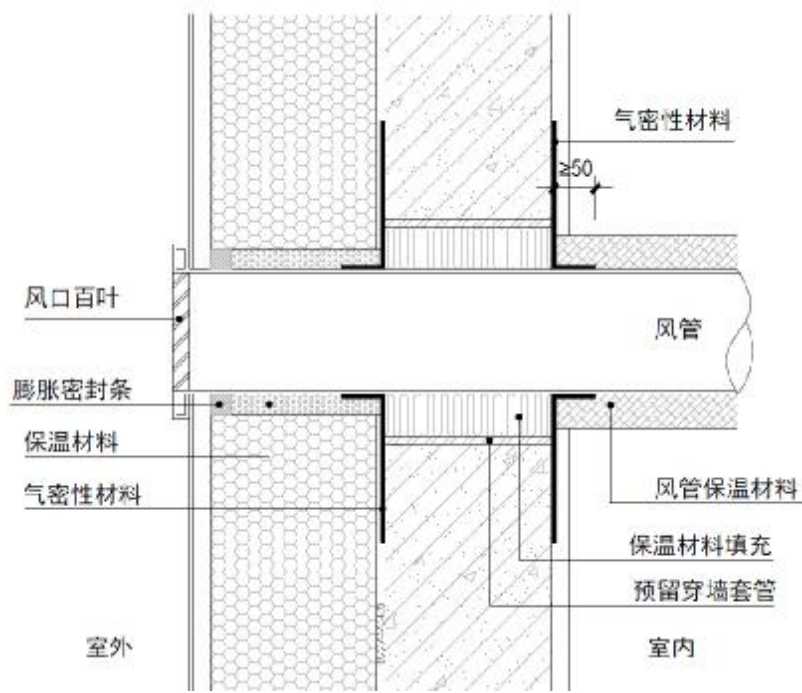
图 7 穿墙风管示意图
