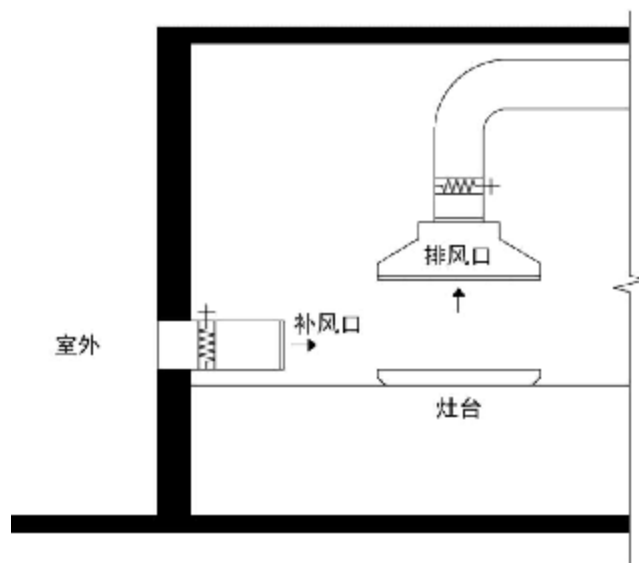
图 19 厨房补风示意图
