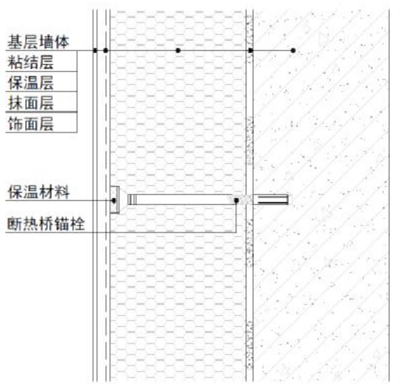
图 5 断热锚栓安装示意图
