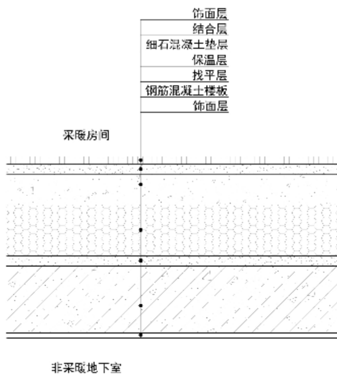
图 13 非采暖地下室顶板保温构造示意图 1
