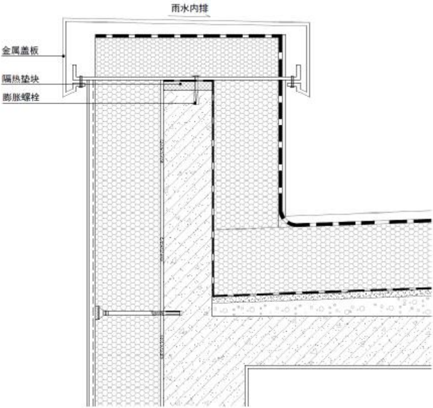
图 10 突出屋面女儿墙及盖板保温构造示意图
