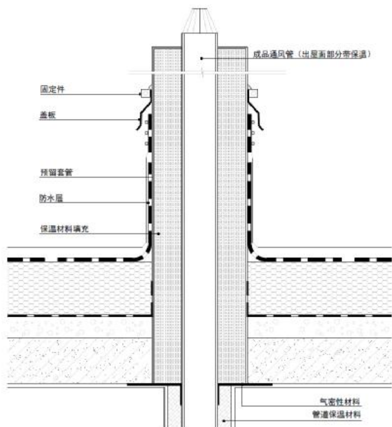
图 12 落水管示意图
