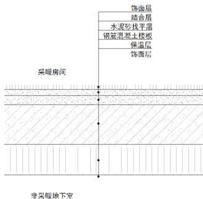
图 14 非采暖地下室顶板保温构造示意图 2
