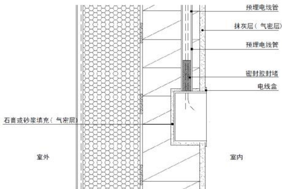
图 17 电线盒气密性处理示意图
