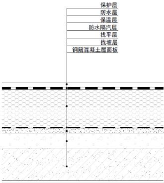
图 9 屋面保温构造示意图
