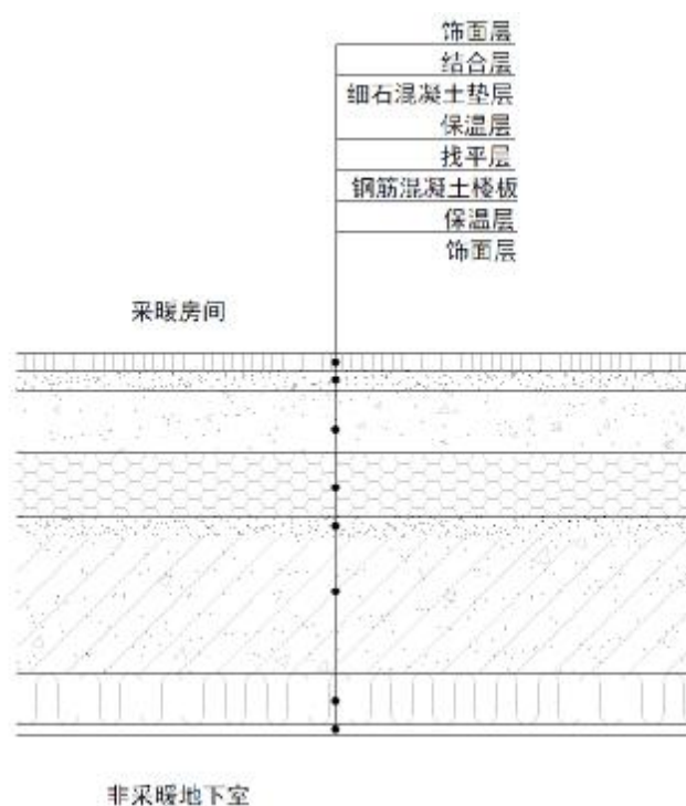
图 15 非采暖地下室顶板保温构造示意图 3
