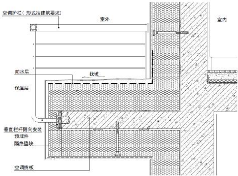
图 6 空调板安装示意图
