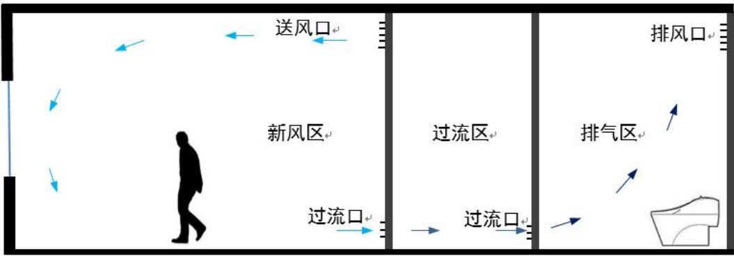
图 18 室内气流示意图
