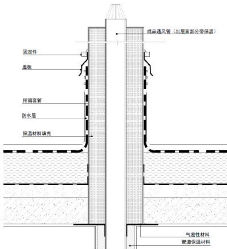
图 11 出屋面管道保温构造示意图
