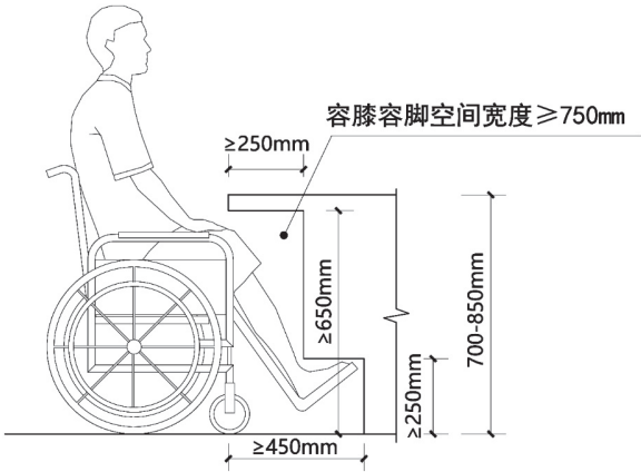
图 5-13 容膝容脚空间示意图
