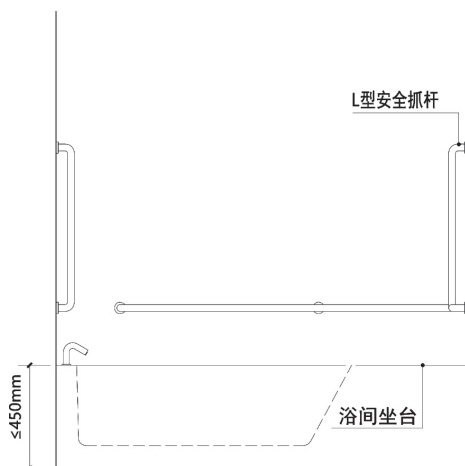
图 5-12 无障碍盆浴间侧立面图
