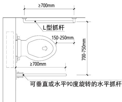
图 5-1 无障碍坐便器 L 型安全抓杆设置平面图
