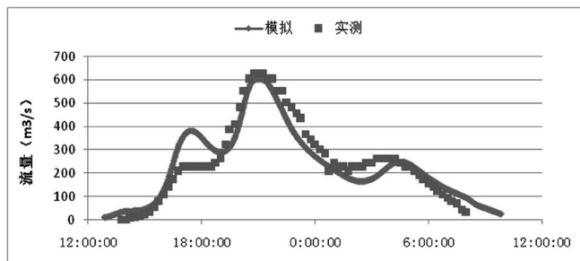
附图 3-2-5-2 清河流域沈家坟断面“7.21”暴雨实测与模拟流量对比图
