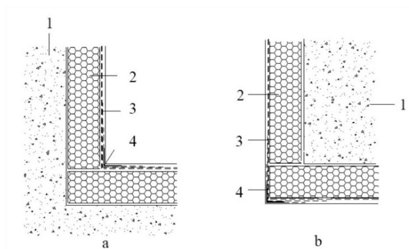
图 7.3.6 阴阳角角网设置示意图
