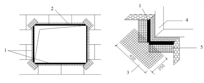
图 7.3.4 门窗洞口耐碱玻璃纤维网布加强图
