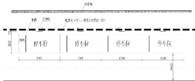
图 A.1-1 “一桩一充”式充电桩平行式停车位的典型设计图
