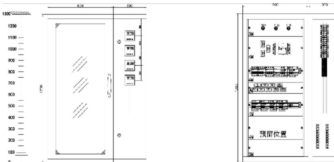
图 6.3.2-2 一种便于监控管理的配电箱基本单元屏面布置示例
