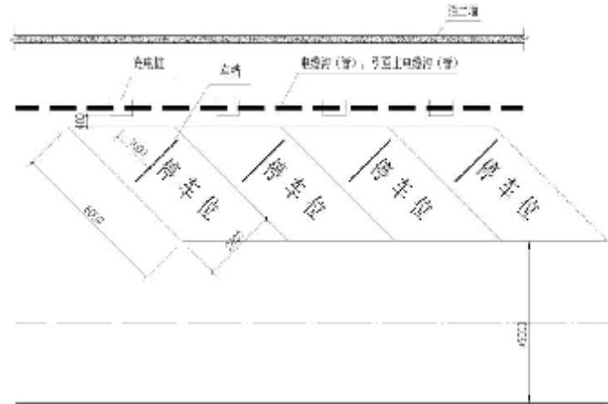
图 A.1-3 “一桩一充”式充电桩倾斜式停车位的典型设计图
