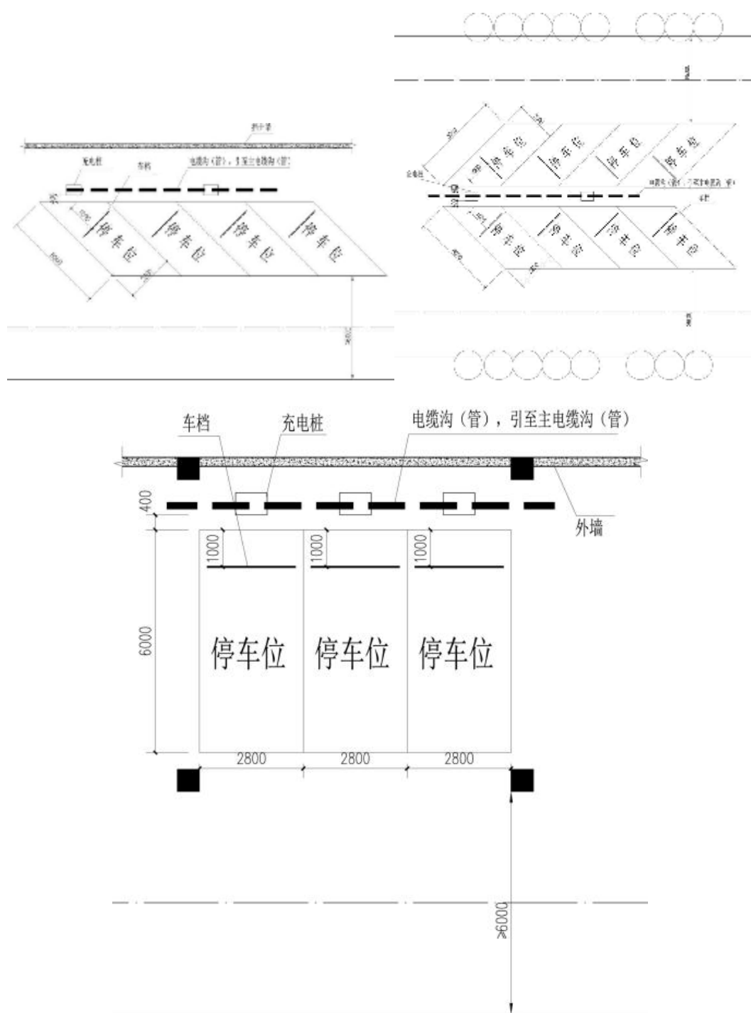
图 A.1-6 “一桩多充”式充电桩倾斜式停车位的典型设计图
