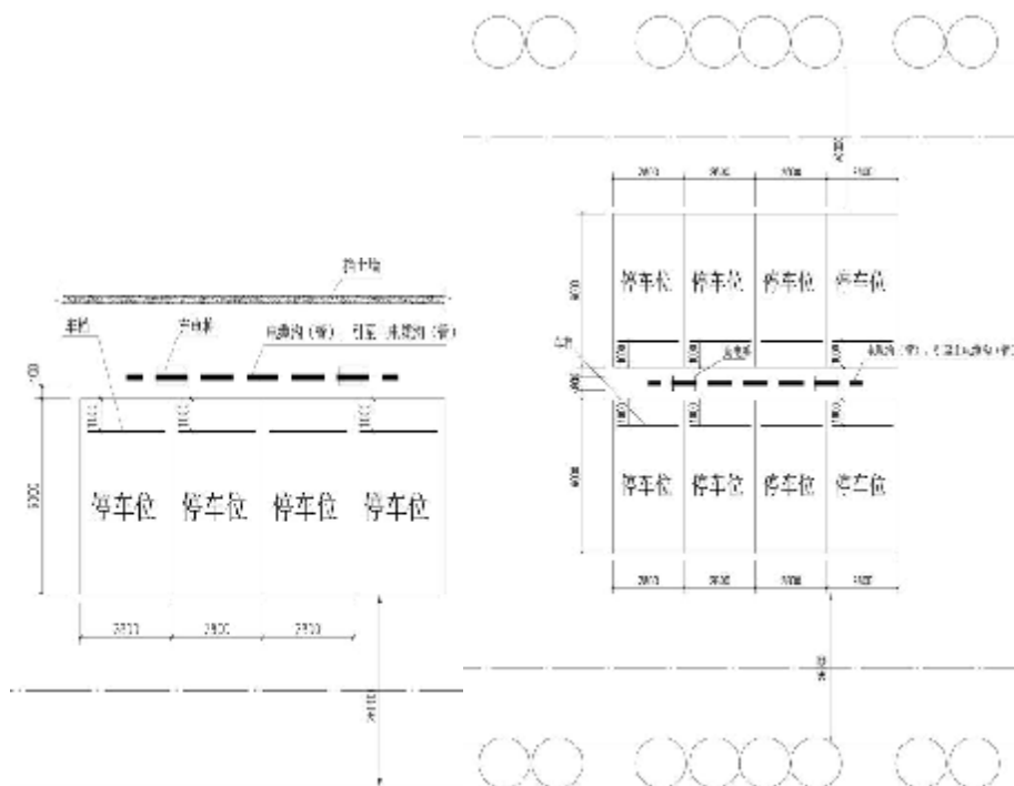
图 A.1-4 “一桩多充”式充电桩平行式停车位的典型设计图
