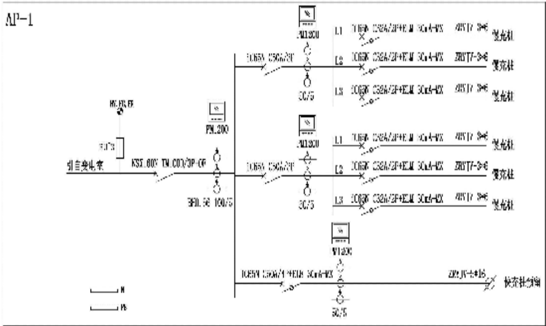
图 6.3.2-1 一种便于监控管理的配电箱基本单元系统示例
