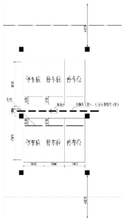
图 A.2-2 “一桩多充”式充电桩垂直式停车位的典型设计图
