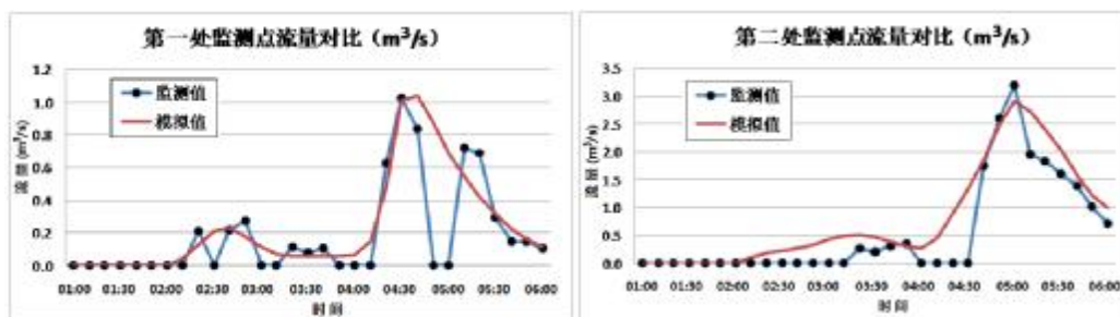
附图 3-1-2-3 2015 年 6 月 26 日 01 点至 06 点管道实测和模拟流量对比图
