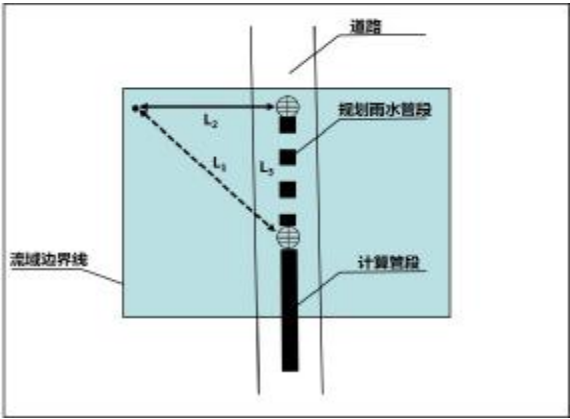
附图 3-2-5-1 地面集水距离示意图
