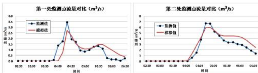
附图 3-1-2-4 2015 年 7 月 18 日 02:30 至 06:30 管道实测和模拟流量对比图
