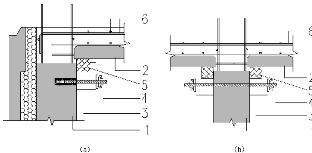
图 15.4.14 叠合板与预制墙板衔接处模板施工节点图
