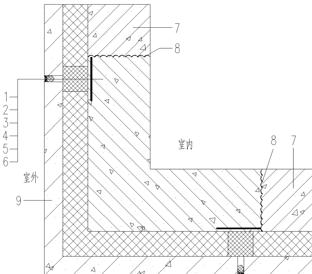
图 15.4.3-2 拐角预制混凝土夹心保温墙板垂直缝密封防水构造
