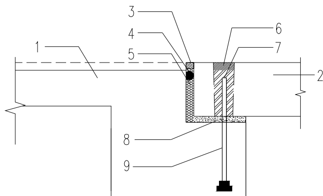
10.4.1 固定铰端安装节点（用于梯段上部）
