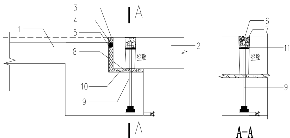
10.4.2 滑动铰端安装节点（用于梯段下部）
