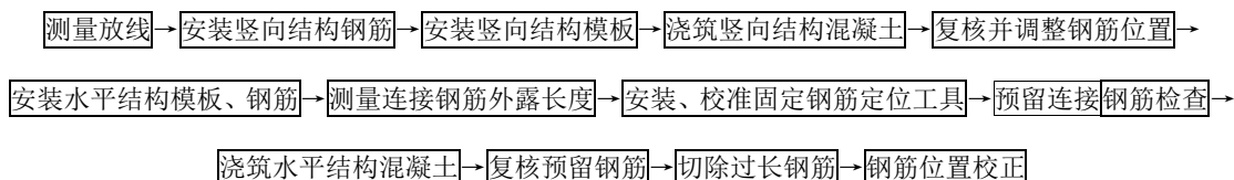
图 3.4.1 转换层施工工艺流程
