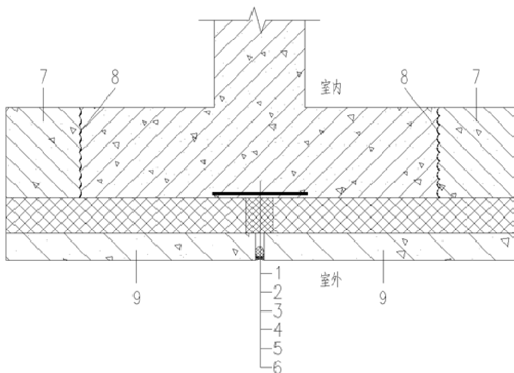
图 15.4.3-1 平直预制混凝土夹心保温墙板垂直缝密封防水构造
