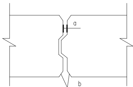
a—弹性密封垫材 ; b—嵌缝槽
