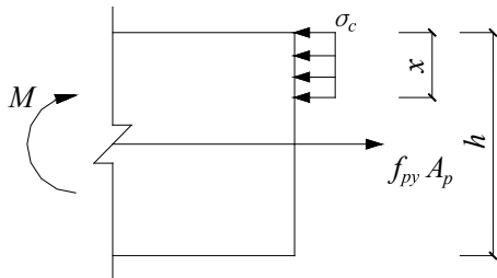
图 6.7.6 接头受弯承载力计算简图
