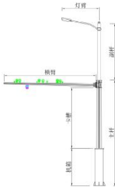
图1 智慧多功能杆杆体组成示意图
