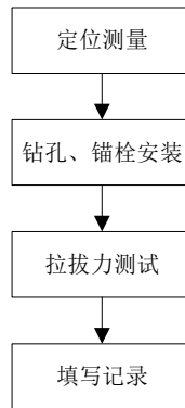
图2 隧道埋入锚栓施工流程
