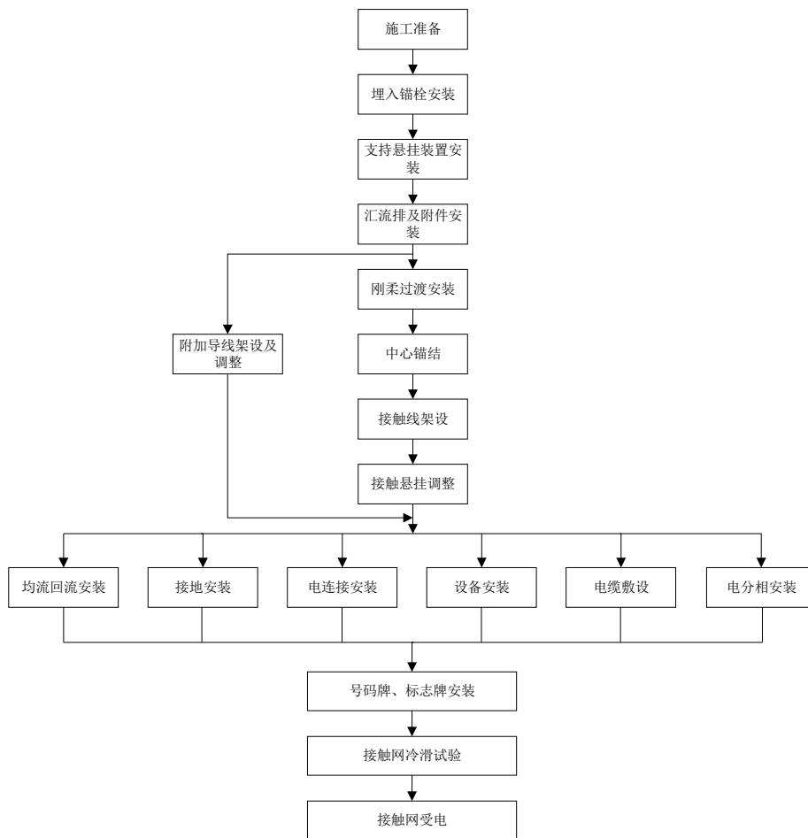
图1 架空刚性接触网施工工序流程
