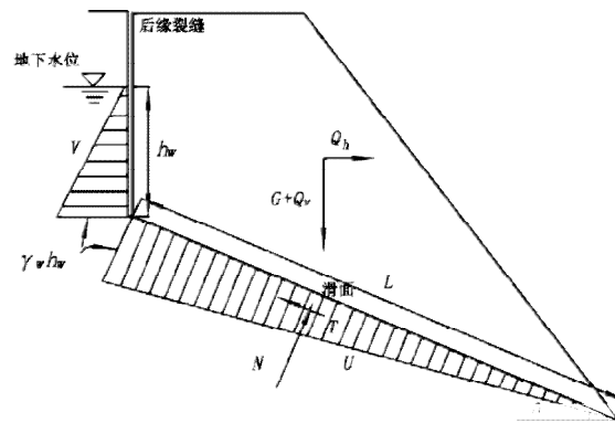
图C.1 后缘有陡倾裂隙且滑面缓倾的滑移式危岩体稳定性计算示意图
