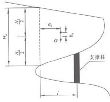
图 M 2 后缘无陡倾裂隙的坠落式剧墙支撑体反力计算示意图
