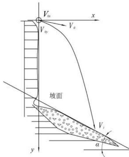
图D.1 危岩体崩落分析模型
