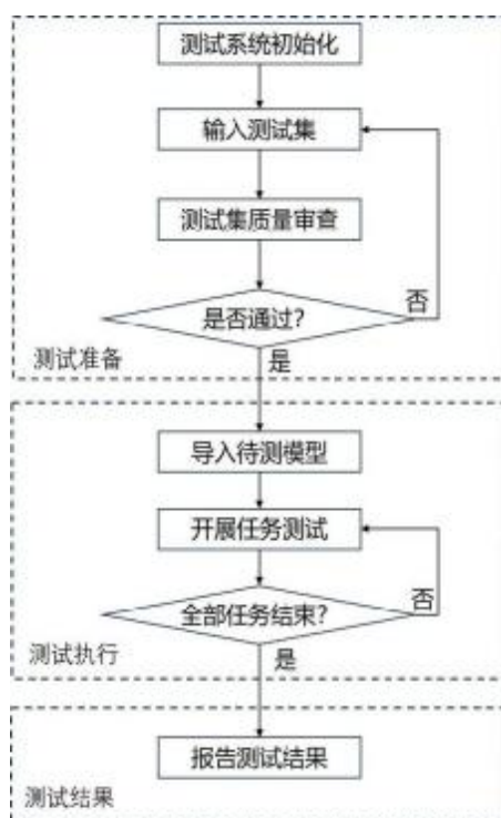
图3 通用人工智能视觉心智能力测试流程
